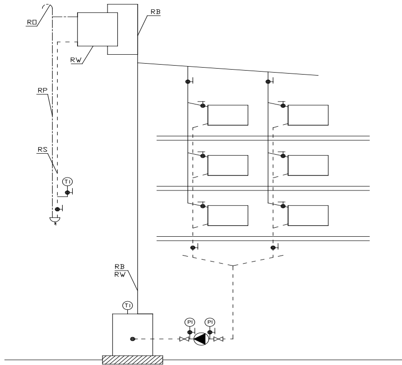
PN-91/B-02413 Schemat zabezpieczenia instalacji ogrzewania wodnego, wyposażonej w jeden kocioł lub wymiennik ciepła, rozdziel górny, pompa zamontowana na powrocie.
