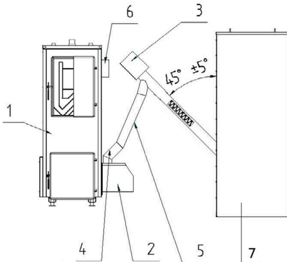
Rys. 1. Zestaw z kotłem Biovert 21 kW
