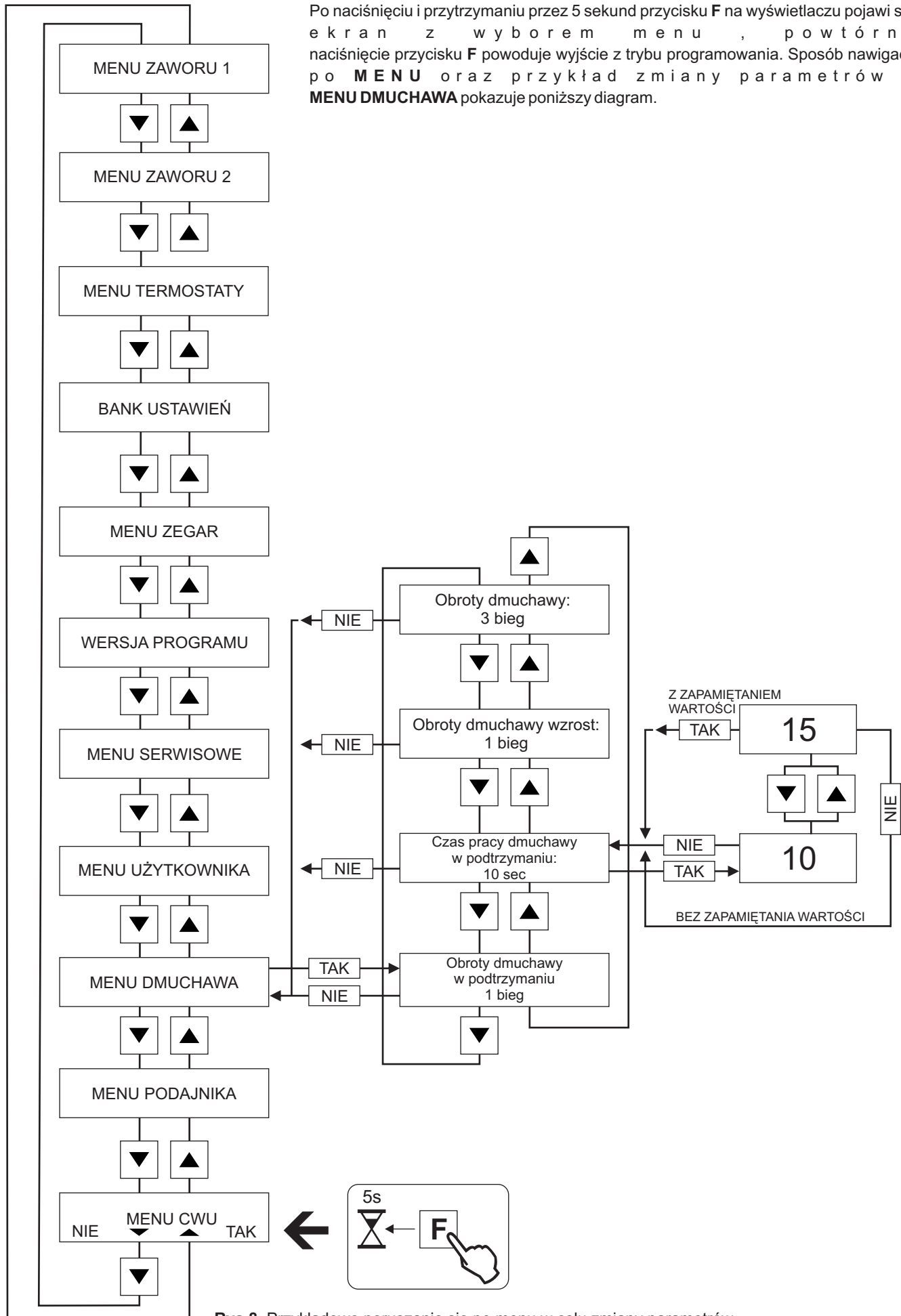
Rys.8. Przykładowe poruszanie się po menu w celu zmiany parametrów
