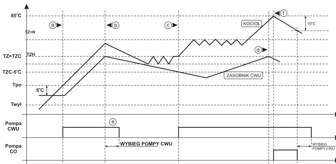
Rys.14. Wykres pracy pompy CO i pompy CWU dla TRYB PRACY CWU=LATO .
